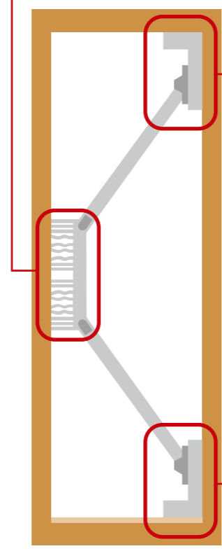
高い減衰性能のアルミデバイス
